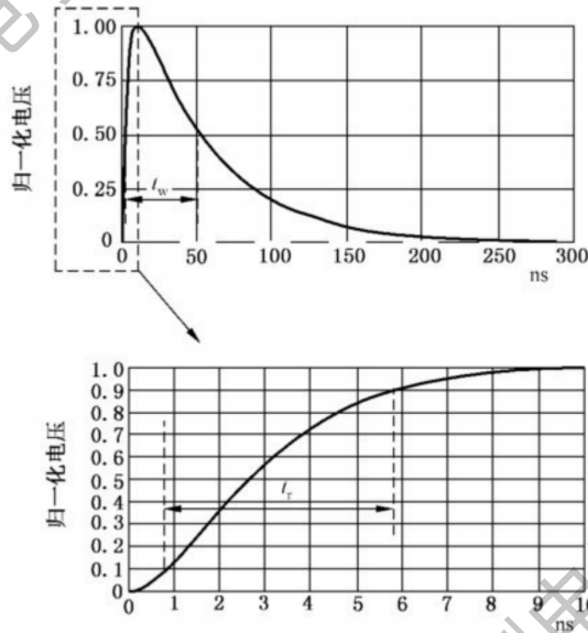
图3 输出到50 Ω负载的单个脉冲的理想波形( t_r=5 ns, t_w=50 ns)
